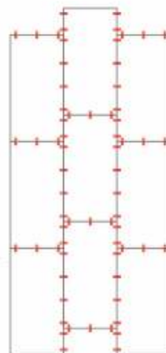
Esquema de instalación de retícula desfasada del formato 60x120 cm
